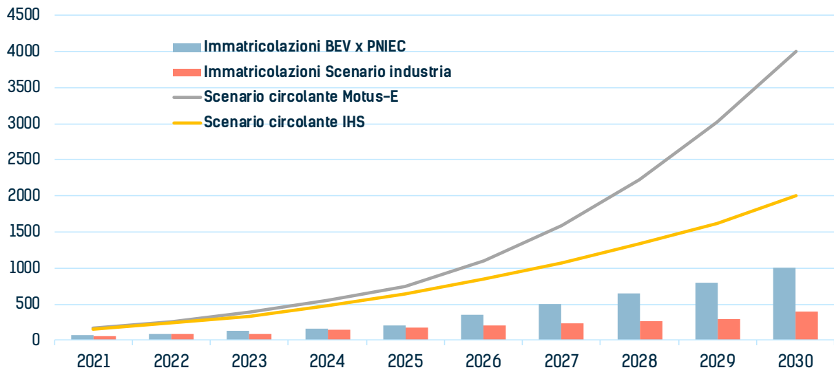
Figura 5.4 Andamenti immatricolazioni e circolante MI BEV
