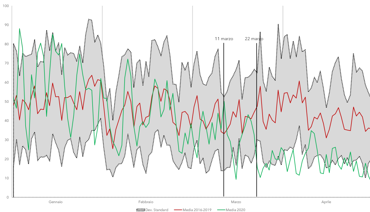
Figura 8 – Napoli: Andamento della concentrazione media giornaliera di \text{NO}_2 nel 2020 e confronto con il periodo 2016-2019 (stazioni di traffico).
