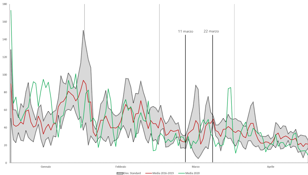
Figura 5 – Milano: Andamento della concentrazione media giornaliera di PM 10 nel 2020 e confronto con il periodo 2016–2019 (stazioni di traffico).
