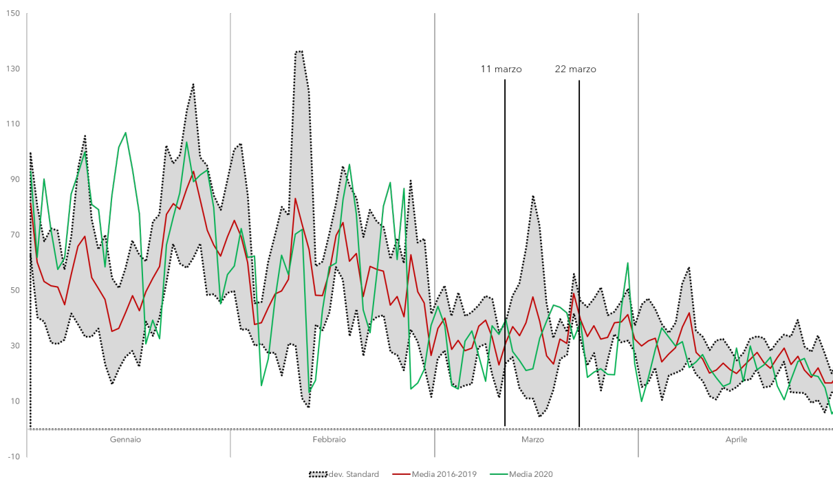
Figura 3 – Torino: Andamento della concentrazione media giornaliera del PM_{10} nel 2020 e confronto con il periodo 2016-2019 (stazioni di traffico).
