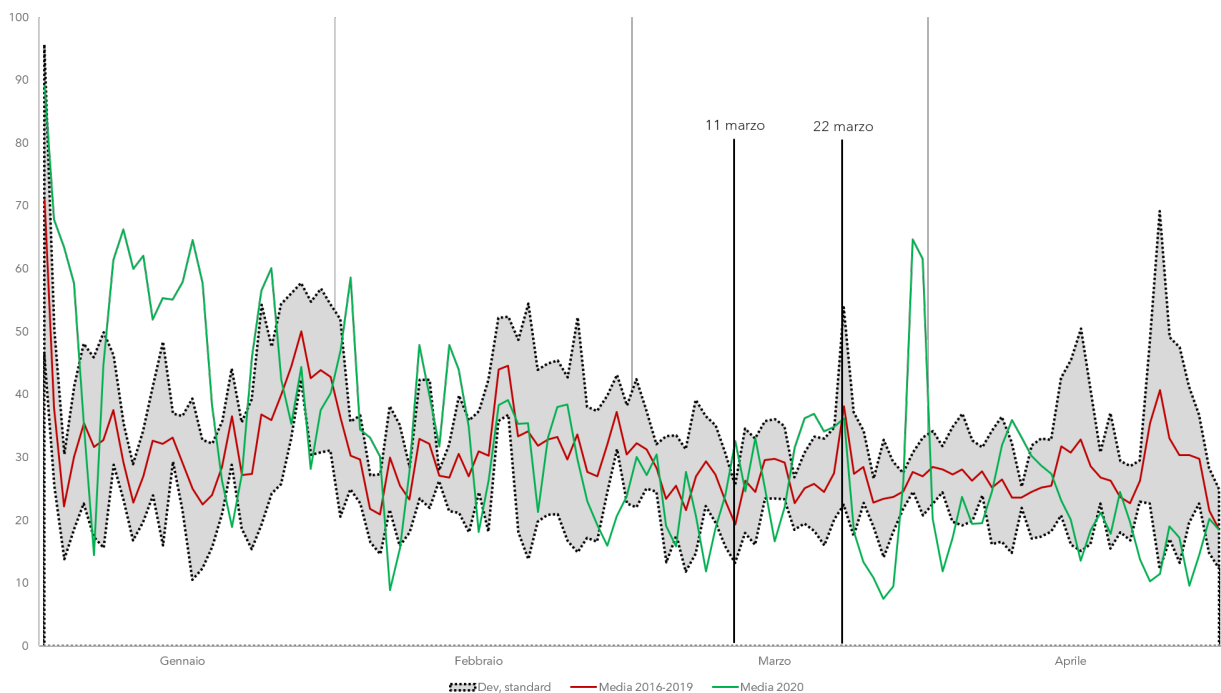
Figura 7 – Roma: Andamento della concentrazione media giornaliera di PM_{10} nel 2020 e confronto con il periodo 2016-2019 (stazioni di traffico).
