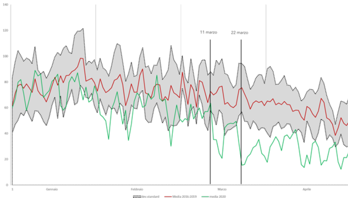
Figura 2 – Torino: Andamento della concentrazione media giornaliera di NO 2 nel 2020 e confronto con il periodo 2016-2019 (stazioni di traffico). La linea rossa indica la media del periodo 2016-2019; l'area in grigio indica la deviazione standard delle misure.
