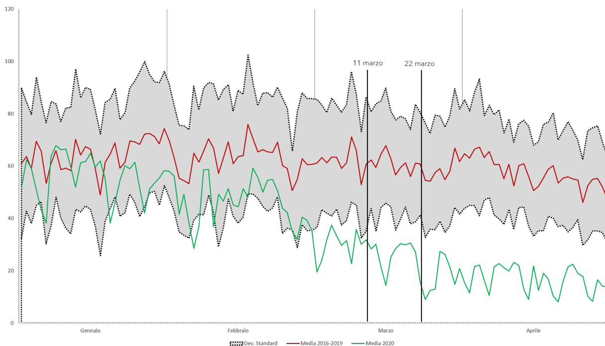
Figura 6 – Roma: Andamento della concentrazione media giornaliera di \text{NO}_2 nel 2020 e confronto con il periodo 2016-2019 (stazioni di traffico).
