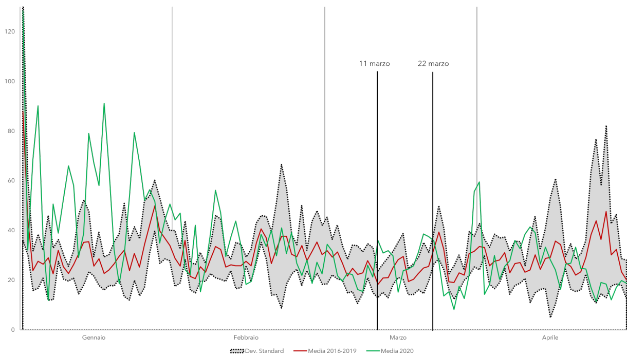
Figura 9 – Napoli: Andamento della concentrazione media giornaliera di PM_{10} nel 2020 e confronto con il periodo 2016-2019 (stazioni di traffico).
