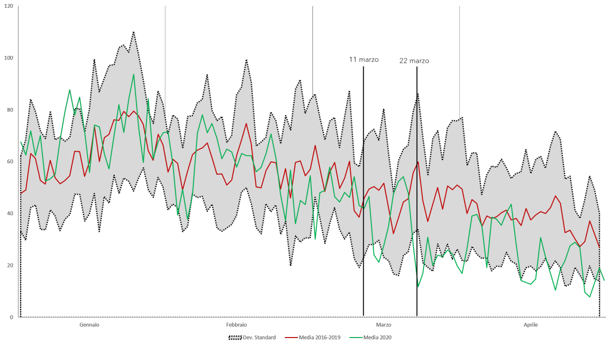
Figura 4 – Milano: Andamento della concentrazione media giornaliera di NO 2 nel 2020 e confronto con il periodo 2016–2019 (stazioni di traffico).
