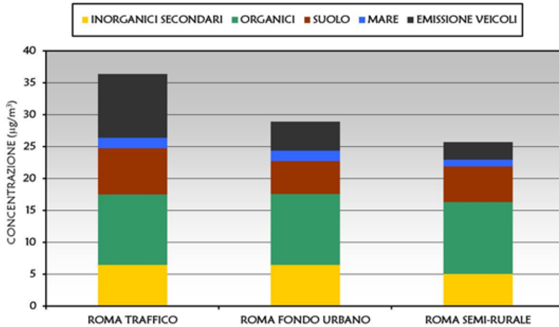
Figura 10 – Composizione media del PM 10 in tre stazioni dell'area urbana e peri-urbana di Roma (anno 2011) 9 .
